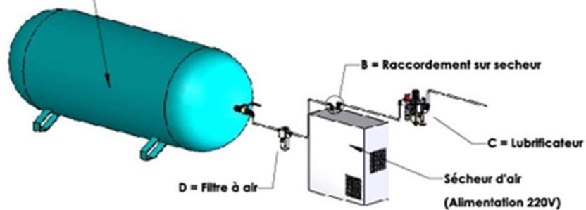
Compresseur 200litres
